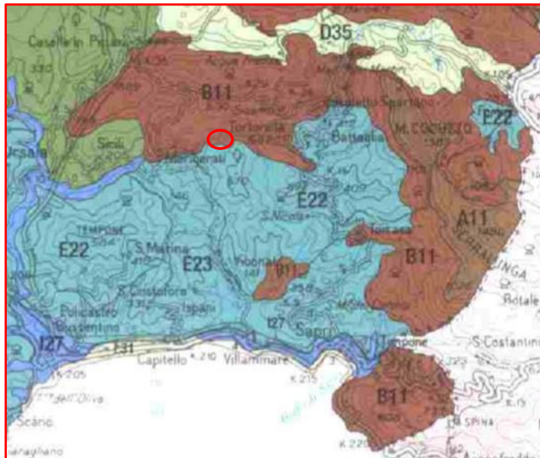
Figura 1 - Stralcio di Carta dei Sistemi di Terra della Campania. In giallo l'area oggetto di studio.
